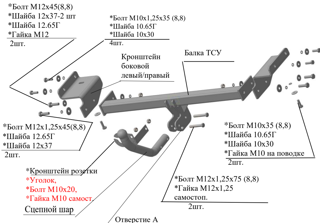
Рис.1 Тягово-сцепное устройство ТСУ 7261.
